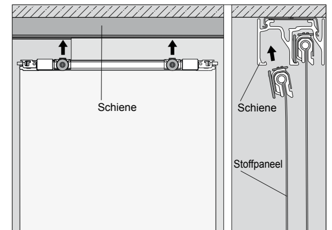
Einfaches Einhängen und Entnehmen des Paneelwagens direkt von unten in die Läufe der Schiene Simple attachment and removal of the panel carrier into the rail runs right from below
